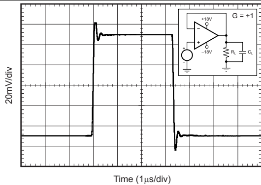
图 15. 小信号过冲与容性负载间的关系
