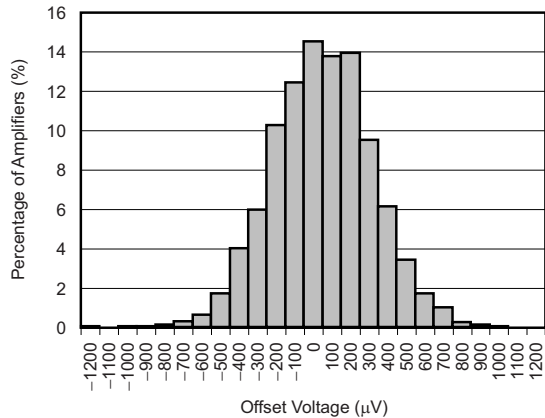
根据 3500 个放大器得出的分布图
