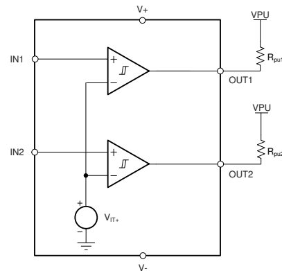
TLV4082-Q1 方框图
