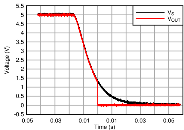
图 8-4. TLV4041/4051 Output for V_S Falling
