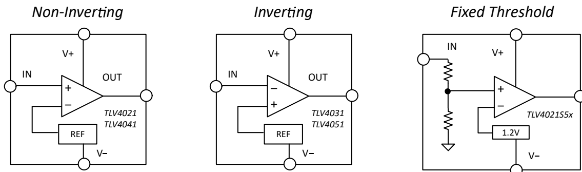
TLV40x1 配置
