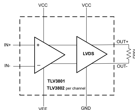
功能方框图
