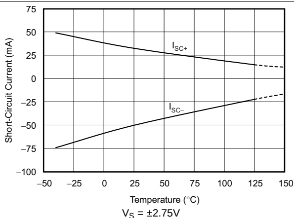
Figure 10. 短路电流与温度间的关系
