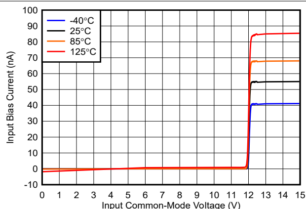
图 6-5. 偏置电流与共模电压间的关系, 12V
