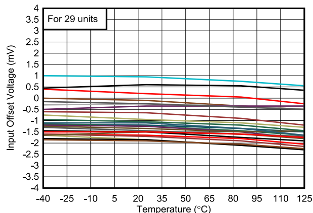
图 6-1. 失调电压与温度间的关系
