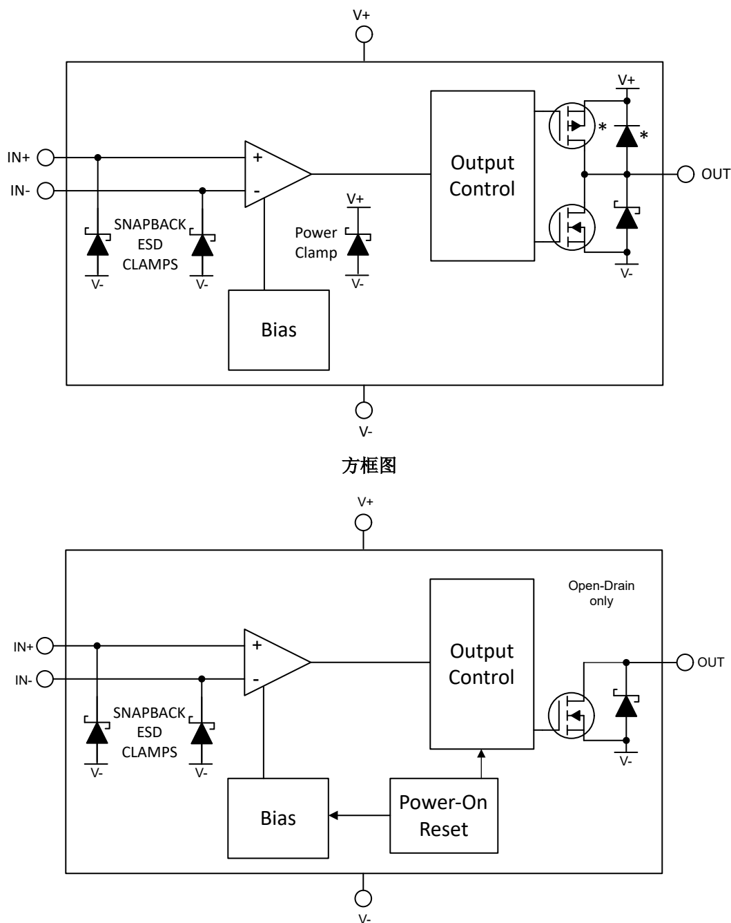
图 7-1. 方框图
