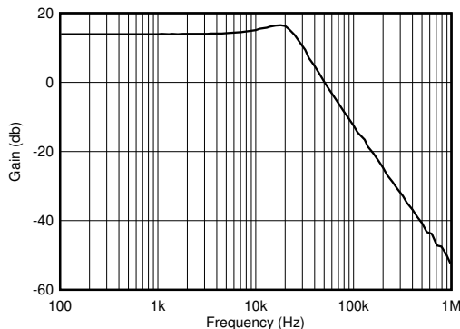
图 8-6. TLVx365 二阶 25kHz 切比雪夫低通滤波器
