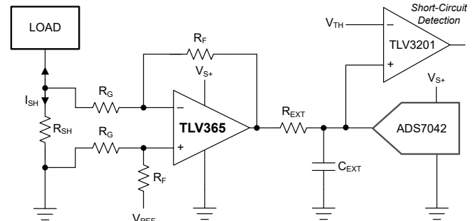
电流检测
