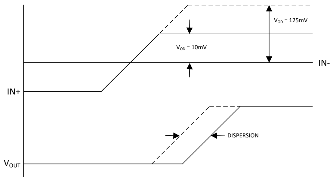
图 6-2. Overdrive Dispersion
