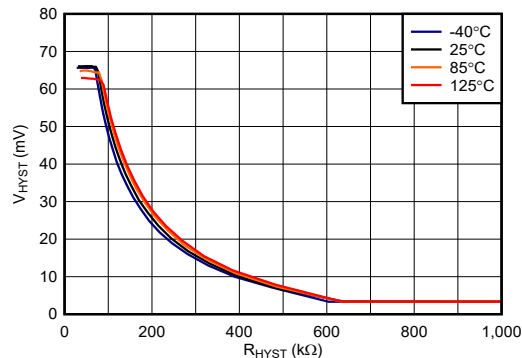
图 8-2. V HYST (mV) vs R HYST (kΩ), V CC = 5 V
