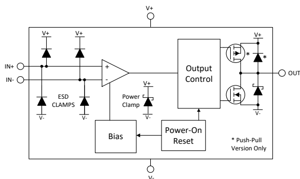
图 6-1. 方框图
