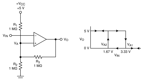
图 7-3. 采用反相配置且具有迟滞功能的 TLV3511-Q1
