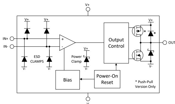
图 6-1. 方框图
