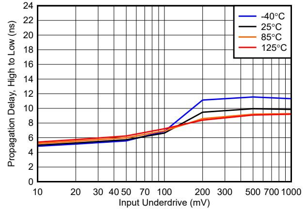
图 5-26. 传播延迟 (高电平到低电平) 与欠驱动间的关系 (5V)
