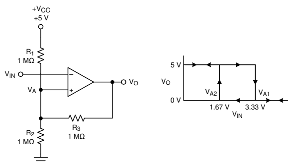
图 7-3. 采用反相配置且具有迟滞功能的 TLV3231-Q1
