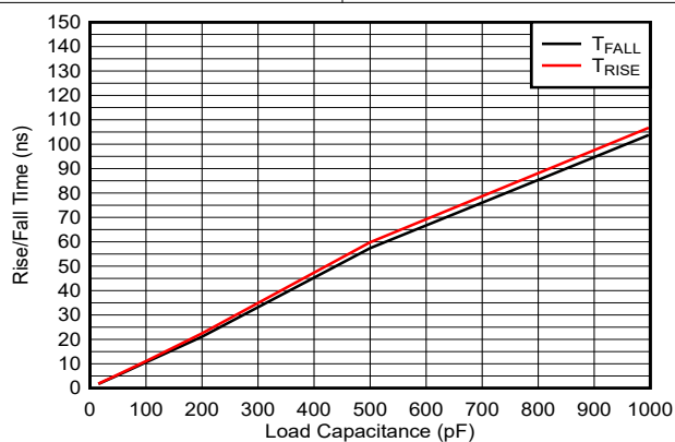
图 5-35. 上升和下降时间与容性负载间的关系
