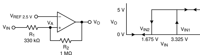
图 7-5. 采用非反相配置、具有迟滞功能的 TLV3231-Q1
