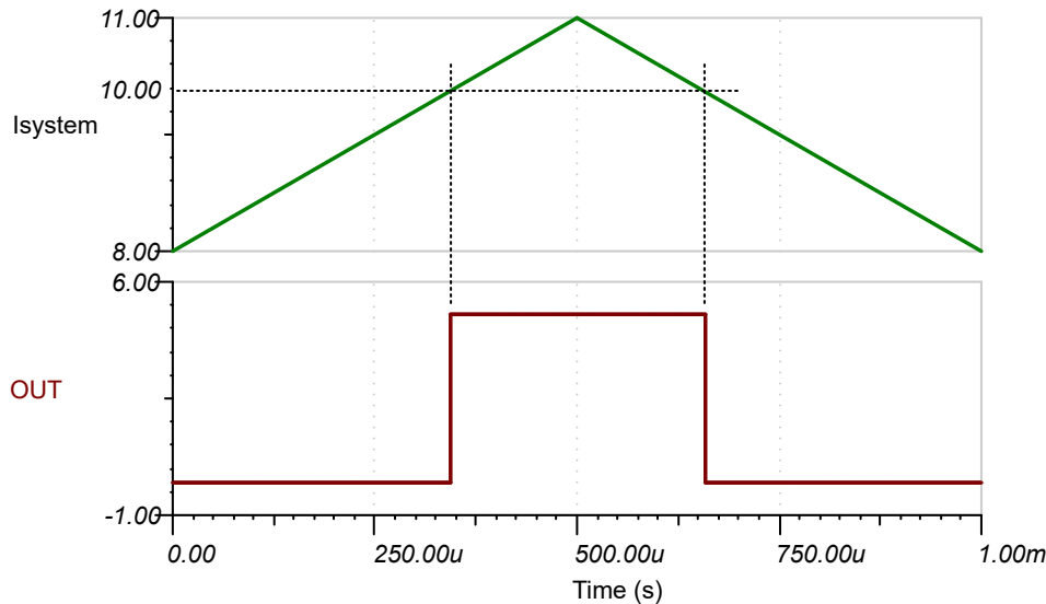
图 7-8. 过流结果
