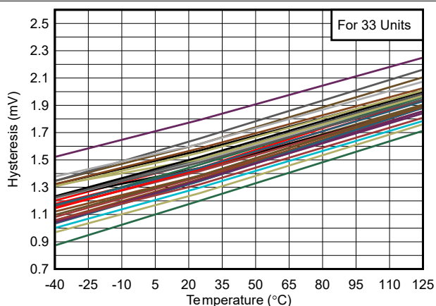
图 5-2. 迟滞与温度之间的关系
