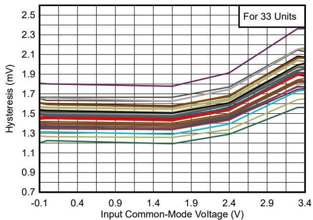
图 5-4. 迟滞与共模电压间的关系, 3.3V
