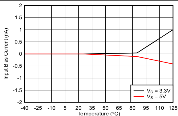
图 5-8. 偏置电流与温度间的关系
