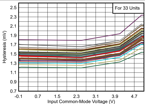
图 5-6. 迟滞与共模电压间的关系, 5V
