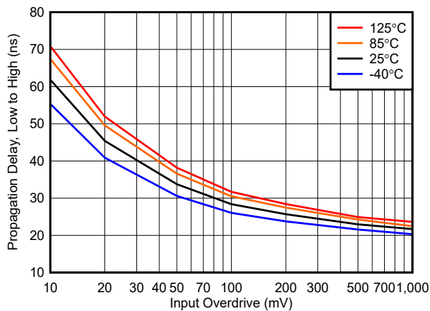
图 5-30. 在 1.8V 时低电平到高电平的传播延迟与过驱间的关系
