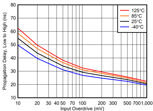
图 5-26. 在 1.8V 时低电平到高电平的传播延迟与过驱间的关系
