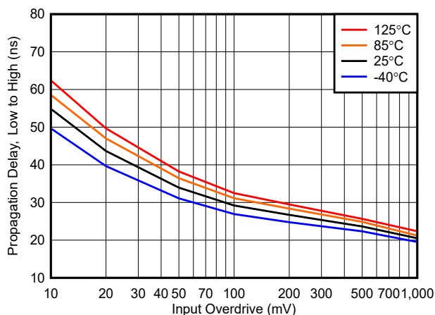
图 5-28. 在 1.8V 时低电平到高电平的传播延迟与过驱间的关系
