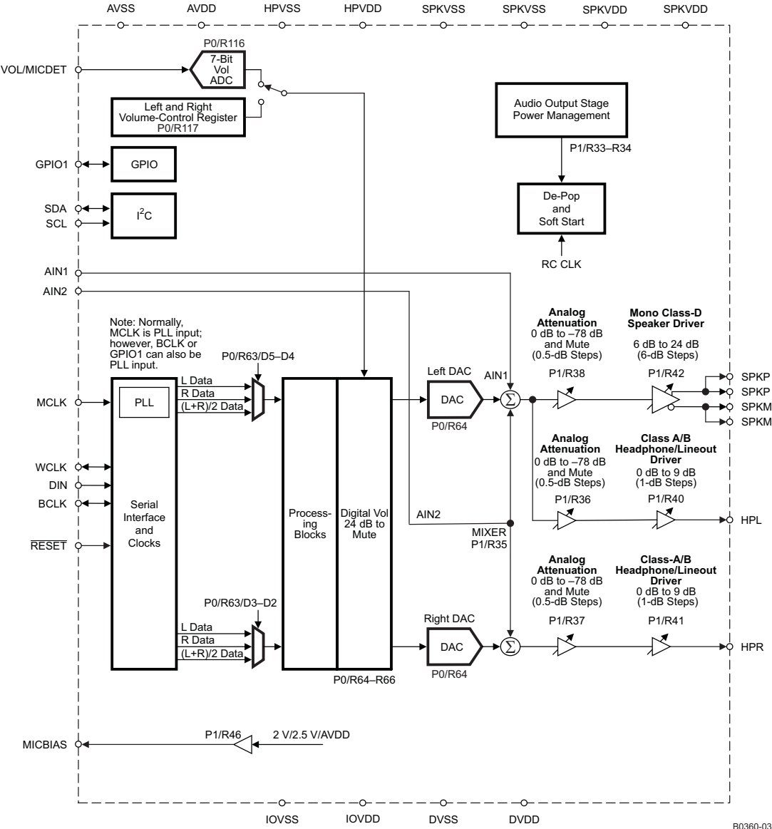
图 1-1. 功能方框图
