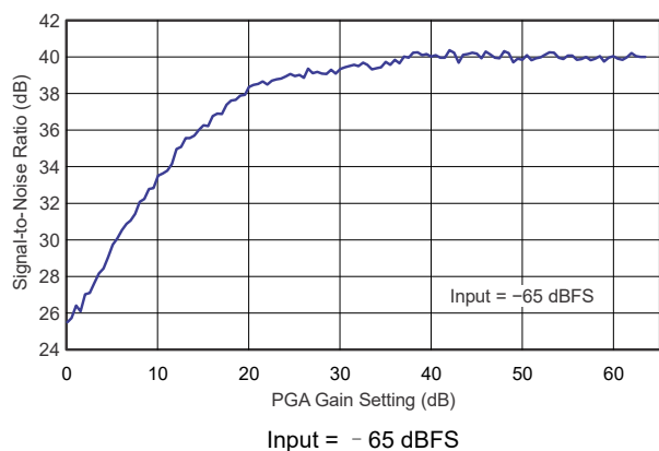
图 6-7. ADC SNR vs PGA Gain Setting, -65-dBFS Input
