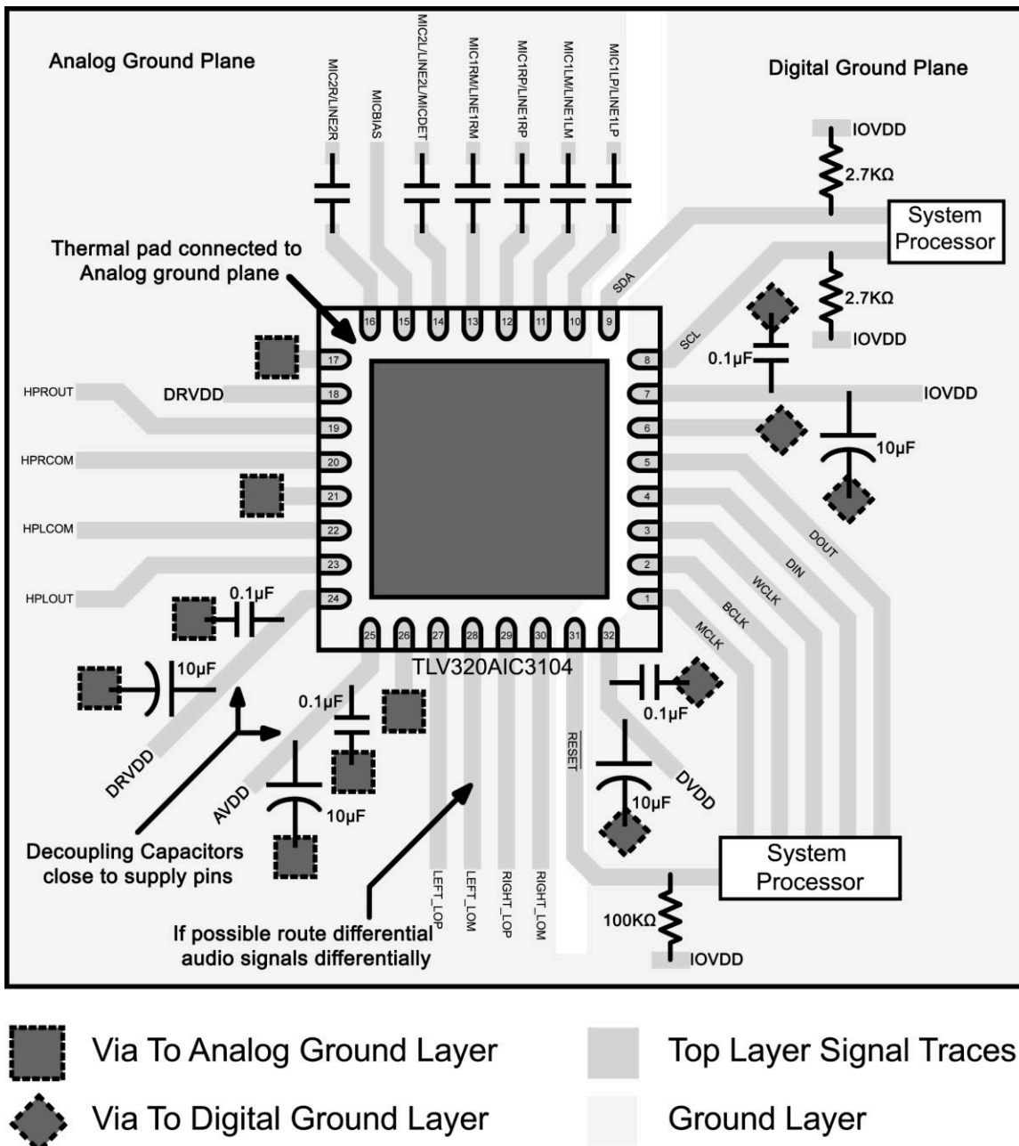
图 13-1. Layout Example
