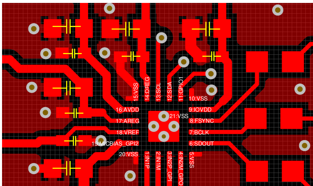
图 11-1. Layout Example
