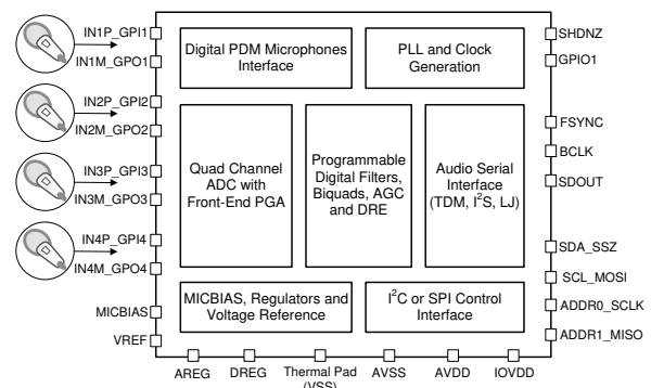
简化方框图
