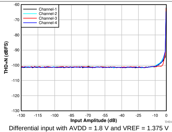
图 7. THD+N vs Input Amplitude
