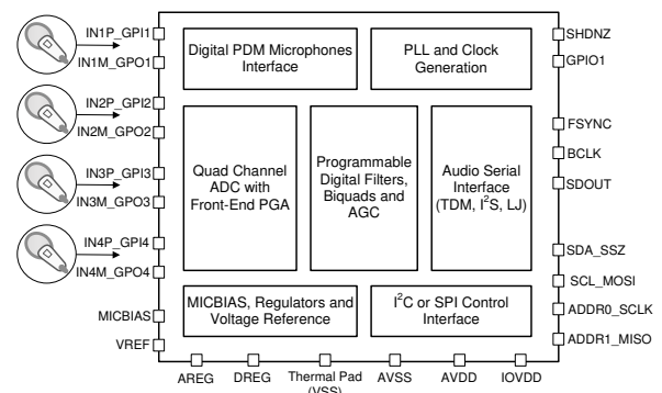
简化方框图
