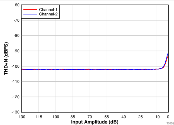
图 7-4. THD+N vs Input Amplitude
