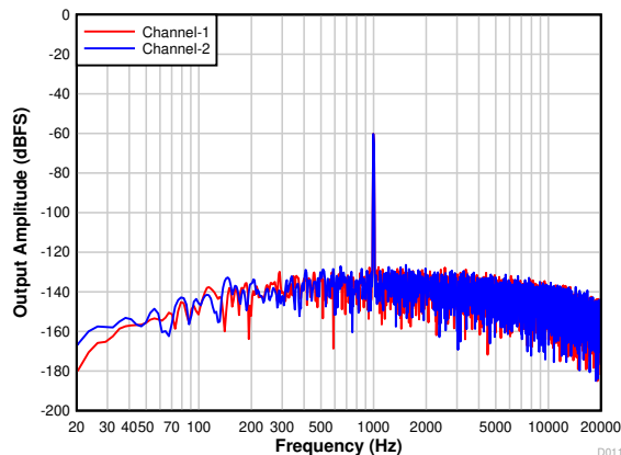
图 7-14. FFT With a -60-dBr Input
