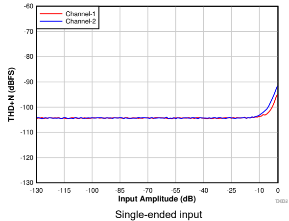
图 7-5. THD+N vs Input Amplitude
