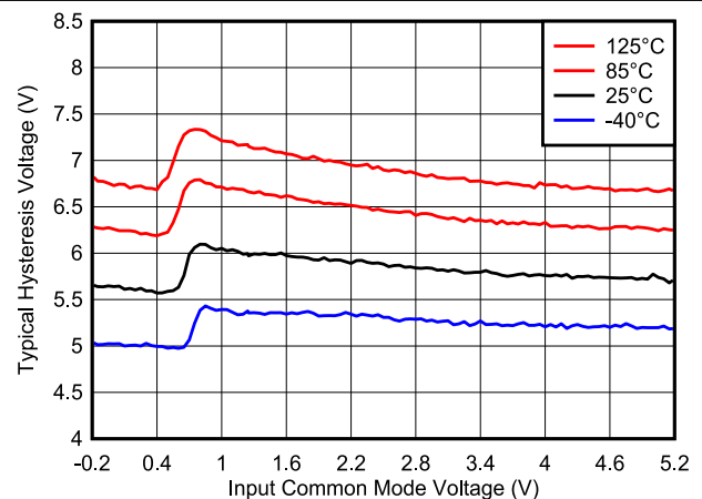
图 6-24. 迟滞电压与共模间的关系, 5\text{V}
