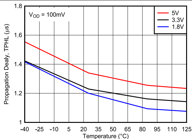
图 6-14. 从高电平到低电平传播延迟时间与温度间的关系
