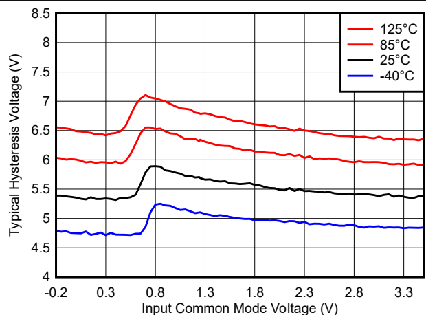
图 6-23. 迟滞电压与共模间的关系, 3.3\text{V}
