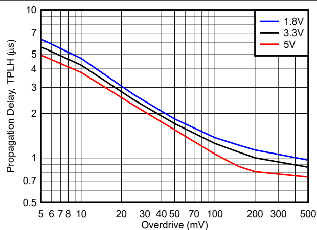
图 6-13. 从低电平到高电平传播延迟时间与过驱动间的关系
