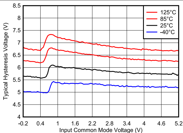
图 6-24. 迟滞电压与共模间的关系, 5\text{V}
