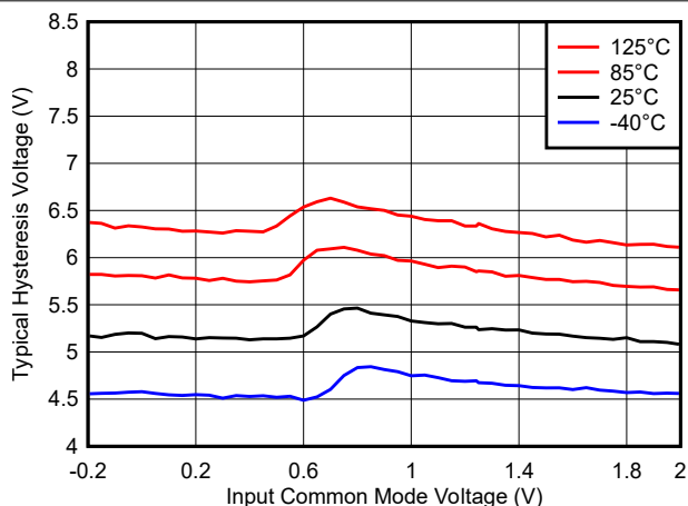
图 6-22. 迟滞电压与共模间的关系, 1.8\text{V}
