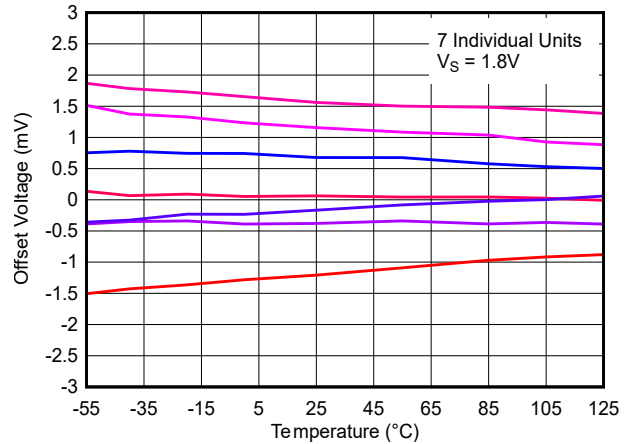
图 6-26. 失调电压与温度间的关系, 1.8V
