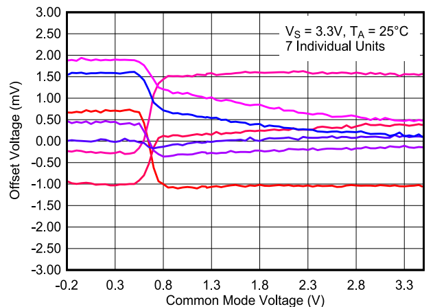
图 6-30. 失调电压与共模电压间的关系, 3.3V
