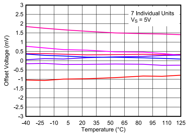
图 6-28. 失调电压与温度间的关系, 5V
