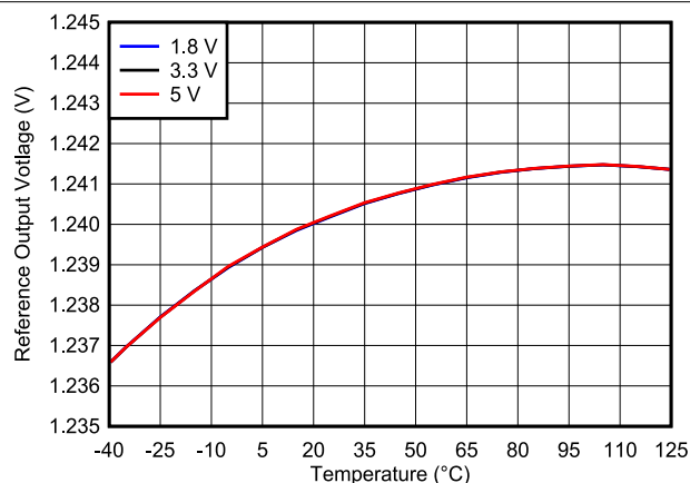
图 6-16. 基准电压与温度间的关系
