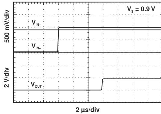
图 7-14. 传播延迟时间 ( t_{PLH} )
