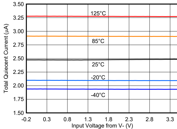
图 8-9. 电源电流与共模间的关系 - 3.3\text{V}
