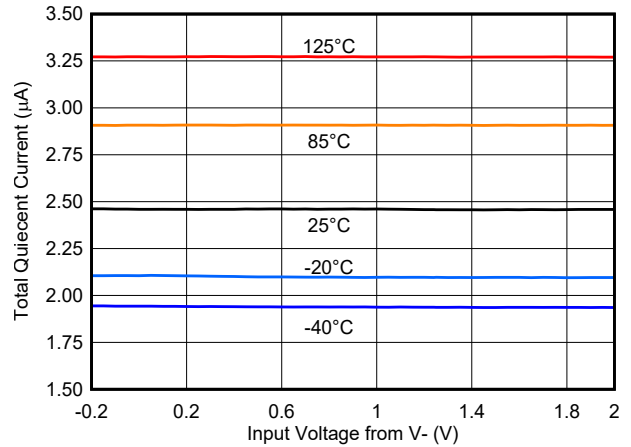
图 8-10. 电源电流与共模间的关系 - 1.8\text{V}
