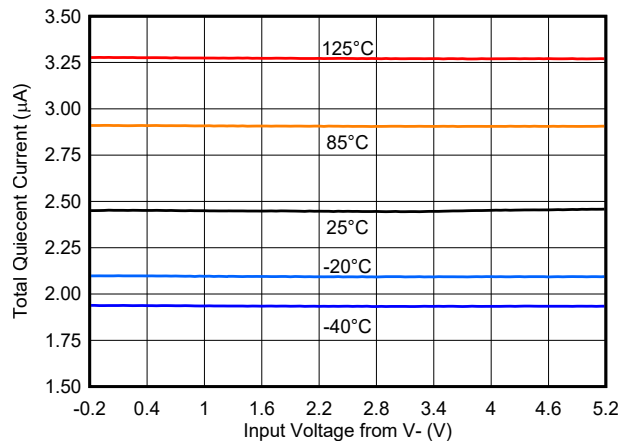
图 8-11. 电源电流与共模间的关系 - 5\text{V}
