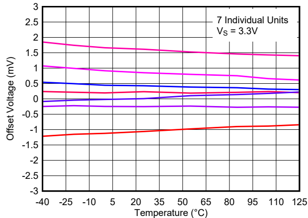
图 8-27. 失调电压与温度间的关系, 3.3V
