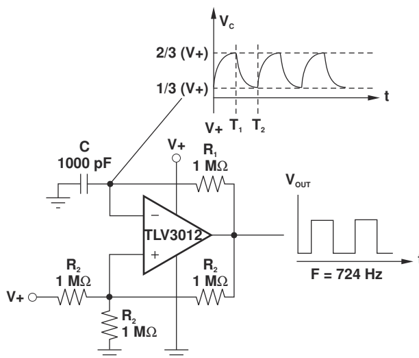
图 10-6. TLV3012 配置为张弛振荡器
