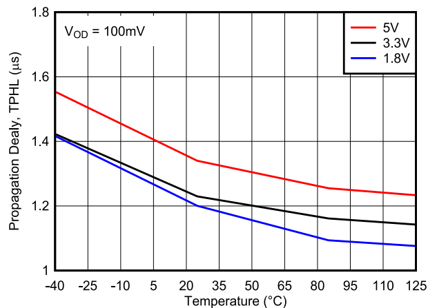
图 8-14. 从高电平到低电平传播延迟时间与温度间的关系
