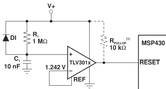
图 10-5. TLV3012 配置为 MSP430™ 微控制器的上电复位电路
