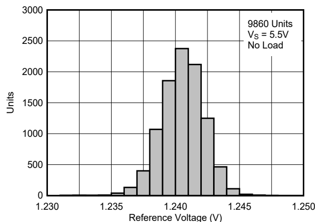
TLV3012B 基准电压分布
