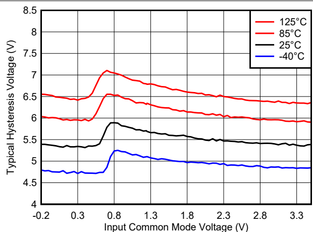
图 8-23. 迟滞电压与共模间的关系, 3.3\text{V}
