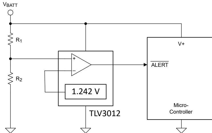
图 10-3. 欠压检测
