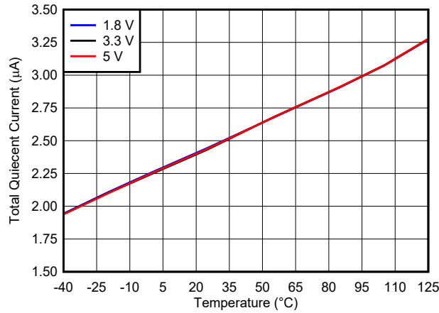
图 8-7. 电源电流与温度间的关系
