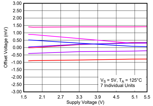
图 8-32. 失调电压与电源电压间的关系, 125°C
