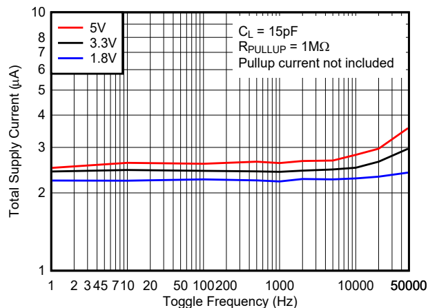
图 8-19. 电源电流与切换频率间的关系 - 开漏输出
