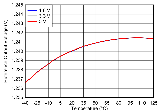
TLV3012B 基准电压与温度间的关系
