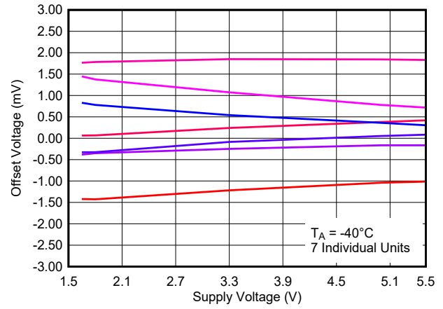
图 8-34. 失调电压与电源电压间的关系, -40°C
