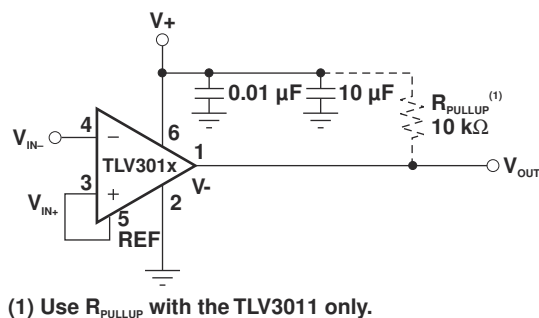
图 10-1. 基本连接
