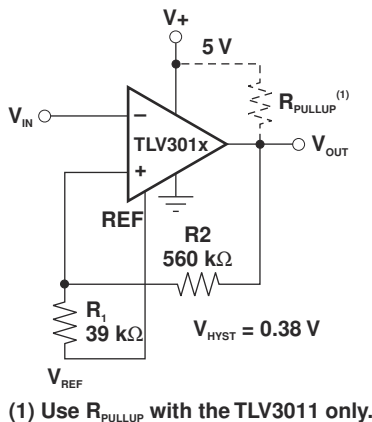
图 10-2. 添加迟滞
