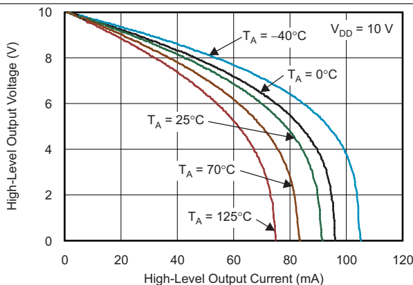
图 6. 高电平输出电压与 高电平输出电流间的关系
