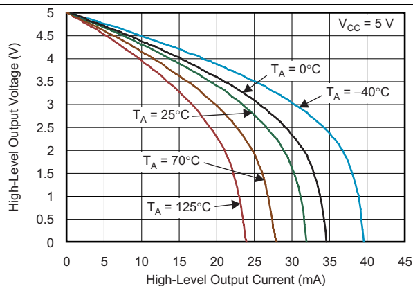
图 4. 高电平输出电压与 高电平输出电流间的关系
