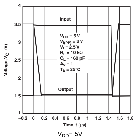
图 45. 反相大信号
