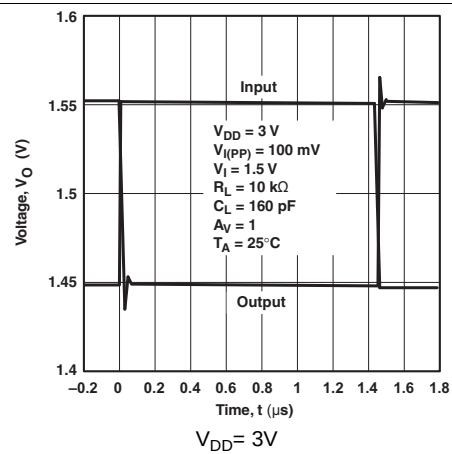
图 46. 反相小信号
