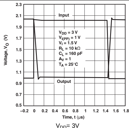
图 44. 反相大信号
