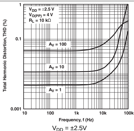
图 33. 总谐波失真与频率间的关系
