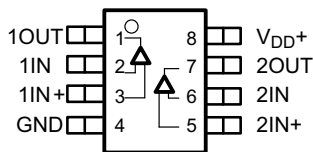
TLV2462-Q1、TLV2462A-Q1 D、DGK 或 PW 封装 8 引脚 SOIC、TSSOP 或 VSSOP 俯视图
