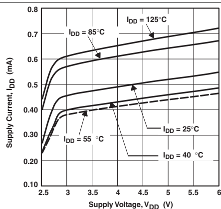
图 20. 电源电流与电源电压间的关系
