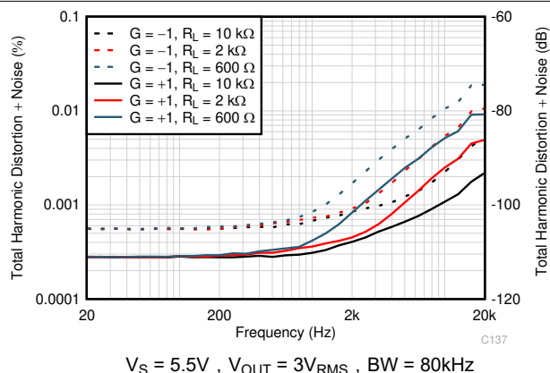
图 5-14. THD+N 比与频率间的关系
