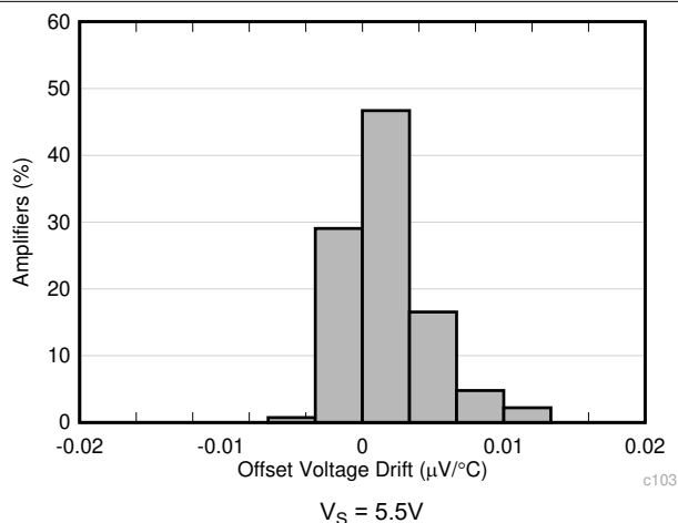
图 5-1. 失调电压温漂分布
