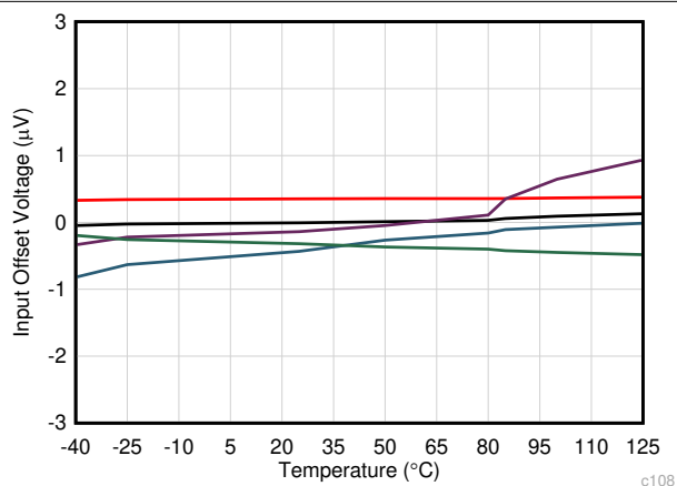
图 5-2. 失调电压与温度之间的关系
