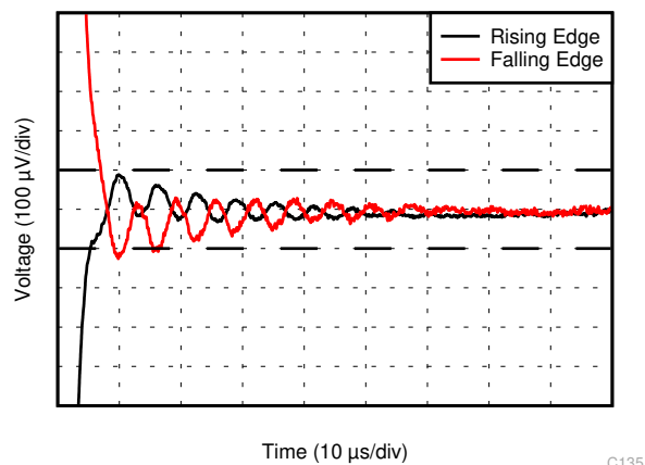
图 5-26. 趋稳时间
