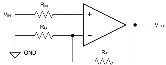
图 7-4. 原理图表示
