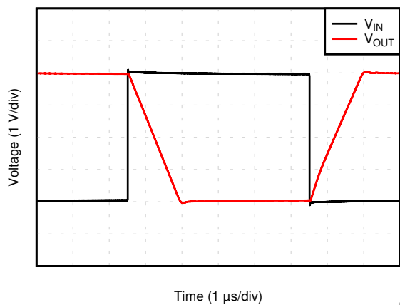
图 5-25. 大信号阶跃响应 (4V 阶跃)
