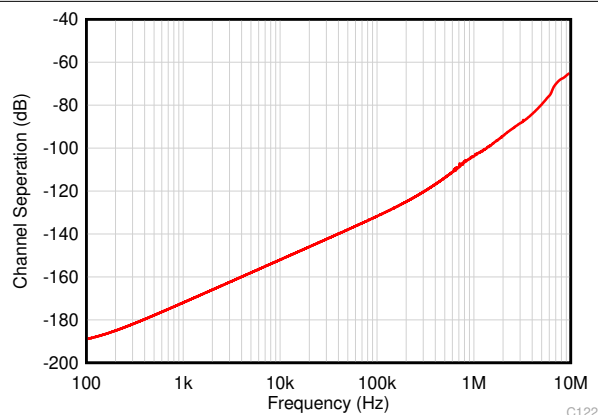
图 5-13. 通道-通道串扰
