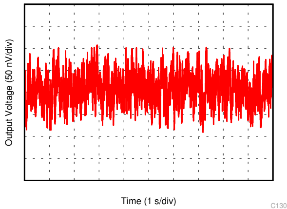
图 5-11. 0.1Hz 至 10Hz 噪声
