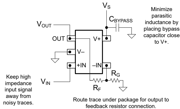
图 7-5. 布局示例
