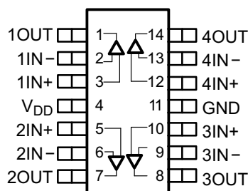
引脚功能: TLV2374-Q1
