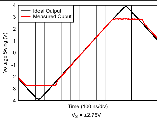
图 6-19. 过驱恢复
