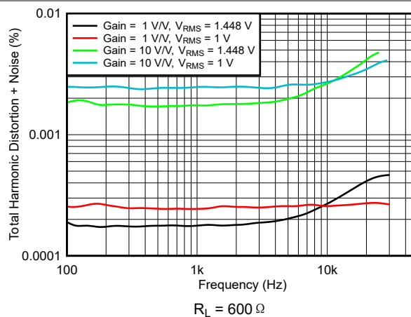
图 6-12. 总谐波失真 + 噪声与频率间的关系
