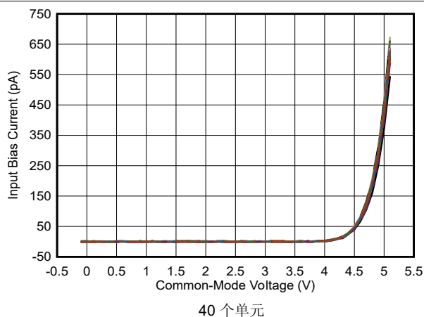
图 6-6. 输入偏置电流与共模电压间的关系
