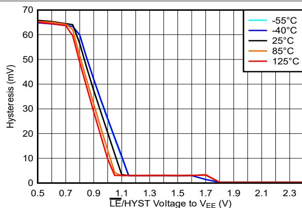
图 5-38. 迟滞电压与 LE/HYST 电压间的关系, 5V
