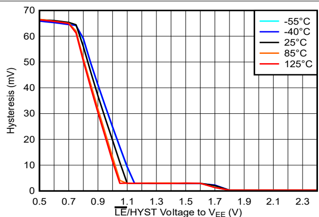
图 5-37. 迟滞电压与 LE/HYST 电压间的关系, 3.3V
