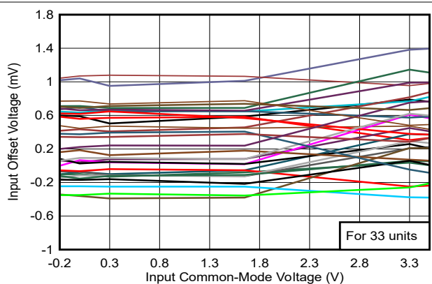
图 5-7. 失调电压与共模电压间的关系，3.3V
