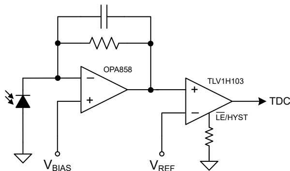
图 7-10. 光学接收器
