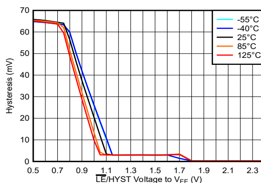
图 7-4. V_{CC} = 5V 时迟滞与 V_{HYS} 间的关系
