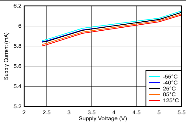
图 5-23. 电源电流与电压间的关系 (输出低电平)
