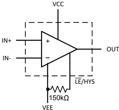
图 7-8. 使用 TLV1H103-SEP 通过电阻器设置迟滞
