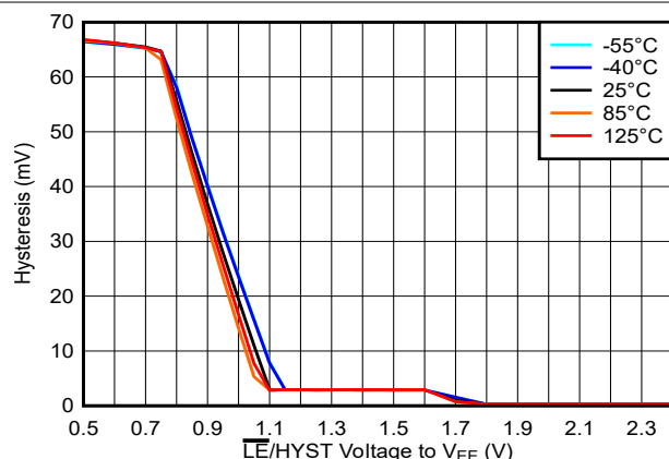
图 5-36. 迟滞电压与 LE/HYST 电压间的关系, 2.5V
