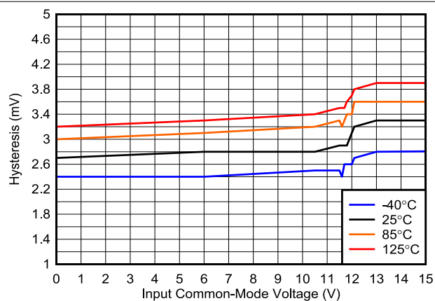
图 6-6. Hysteresis vs. Common-Mode, 12 V
