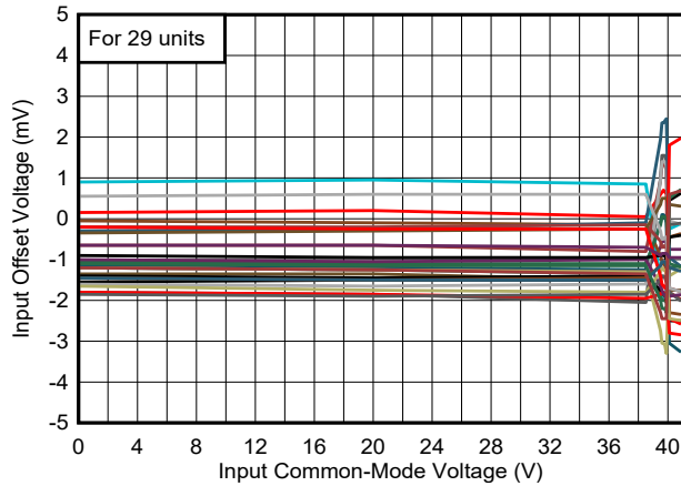
图 6-7. Offset vs. Common-Mode, 40 V
