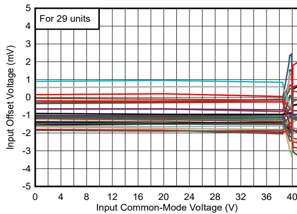
图 5-7. Offset vs. Common-Mode, 40V
