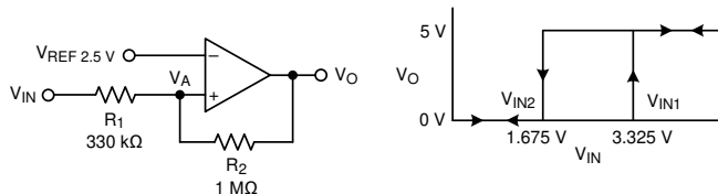
图 7-5. 采用同相配置、具有迟滞功能的 TLV183x-Q1
