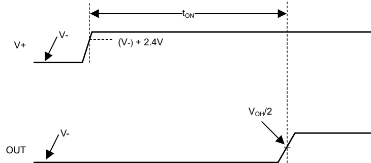
图 7-3. 上电复位时序图
