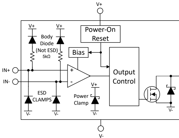
图 7-1. TLV182x 开漏方框图
