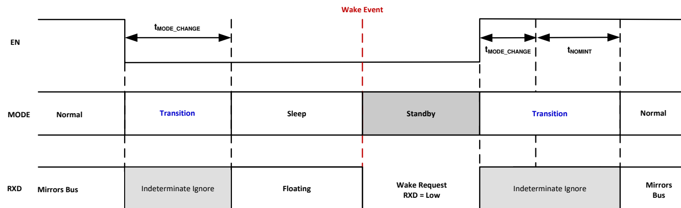
图 8-15. Mode Transitions
