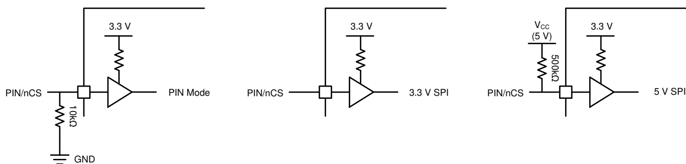
图 9-4. PIN/nCS Configuration
