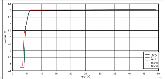
V_{CC} = 5\text{ V} 图 7-6. V_{CC} vs V_{SUP} Across Temperature
