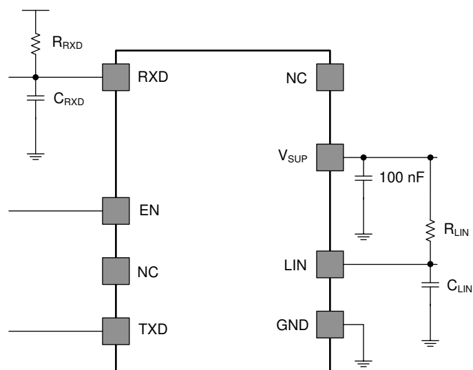
图 6-17. 通过 LIN 唤醒
