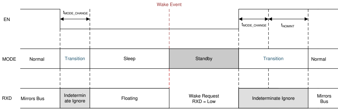
图 8-14. Mode Transitions
