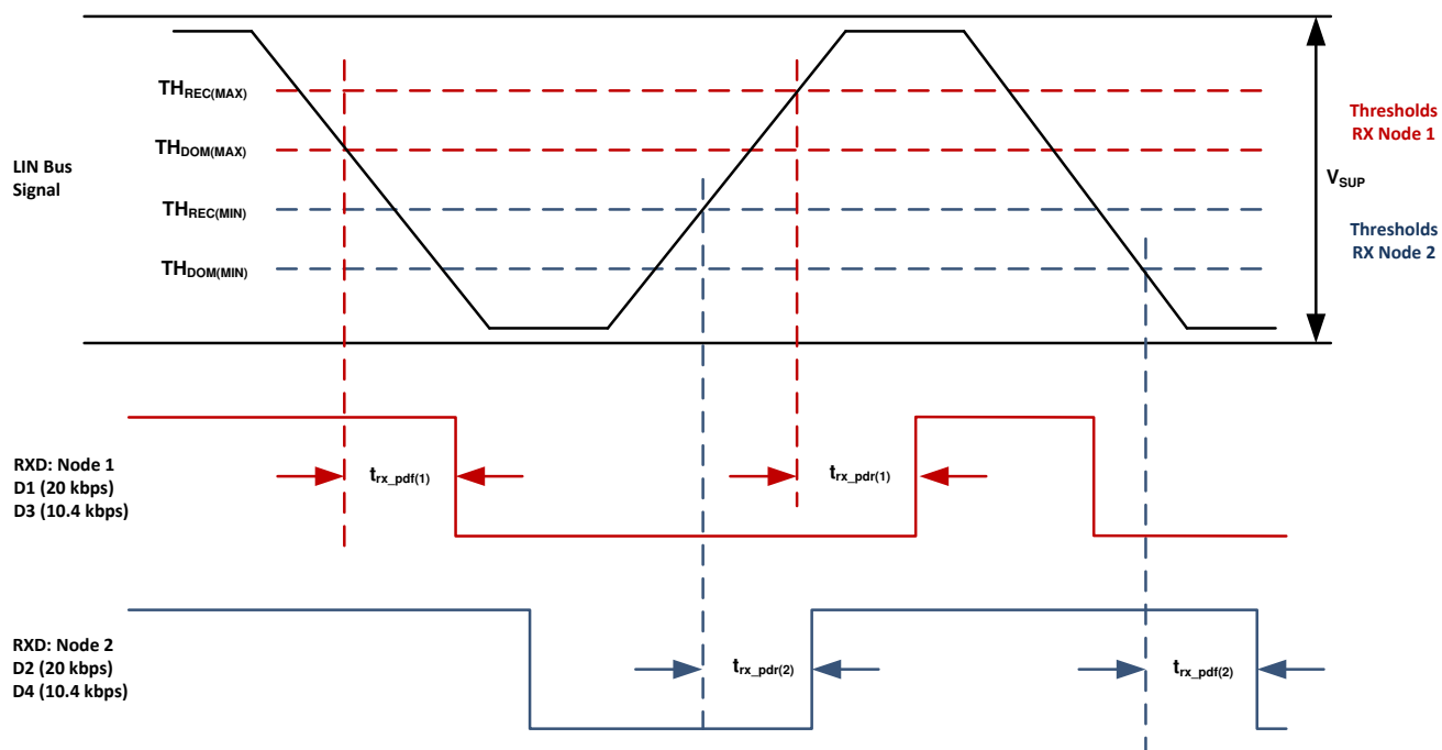
图 8-14. Propagation Delay
