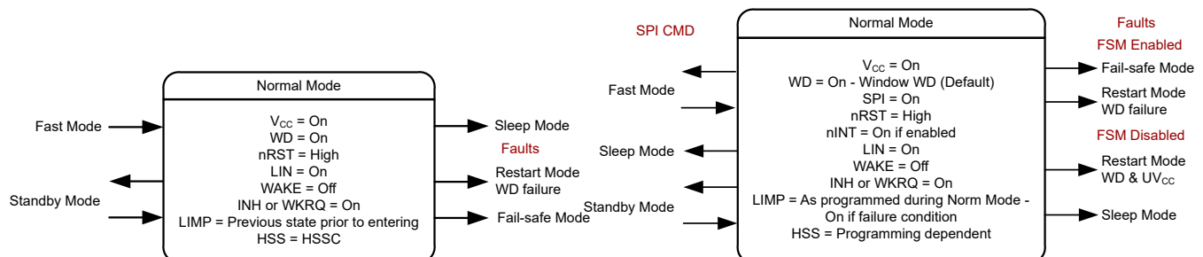
图 8-27. Normal Mode Pin Control
