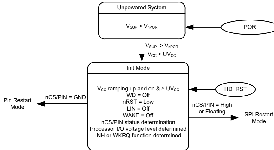
图 8-26. Init Mode
