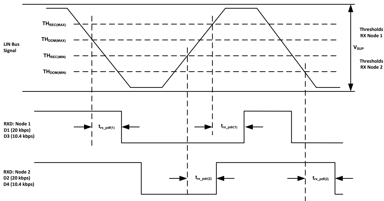
图 7-4. Propagation Delay
