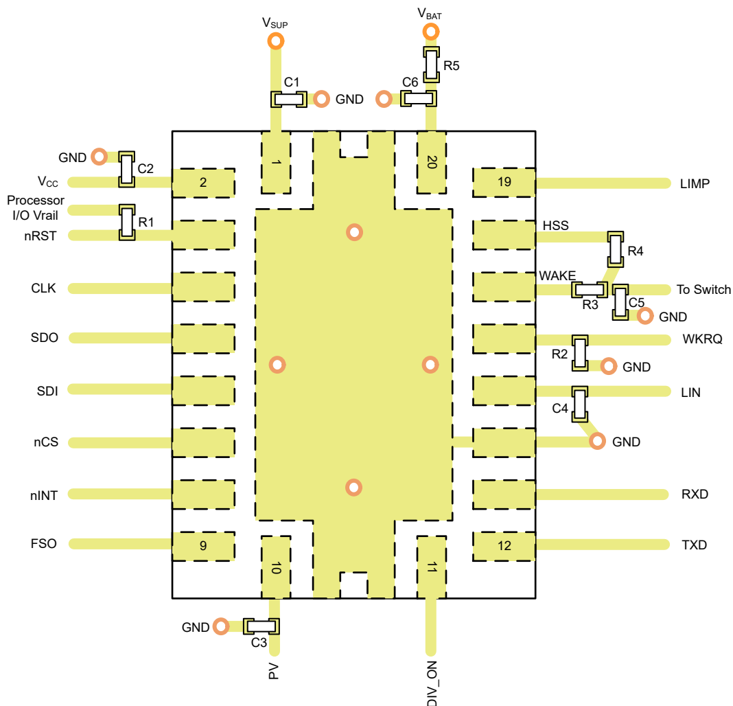
图 9-14. Layout Example
