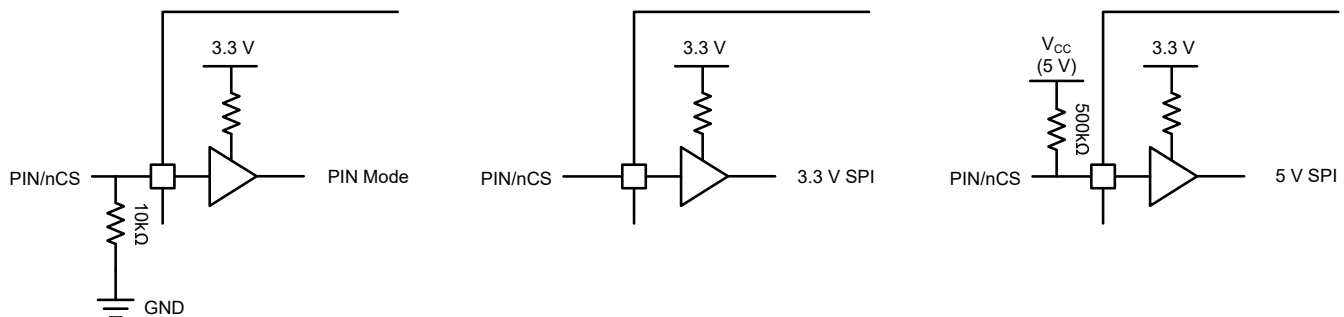
图 8-4. PIN/nCS configuration
