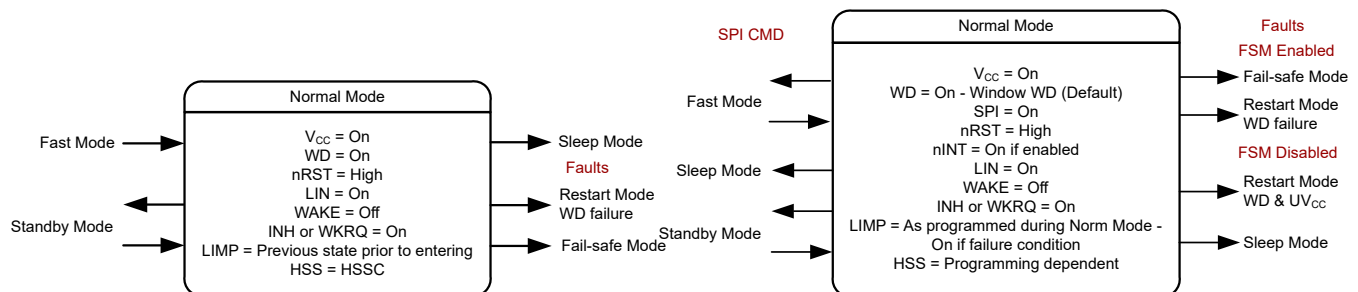
图 8-27. Normal Mode Pin Control
