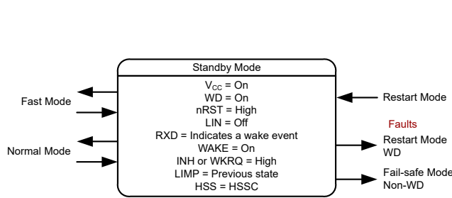
图 8-36. Standby Mode Pin Control
