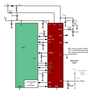
简化版原理图, 引脚控制
