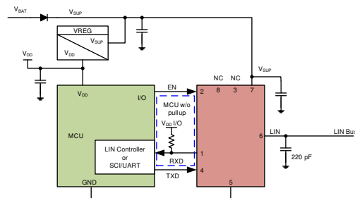
简化版原理图，响应者模式
