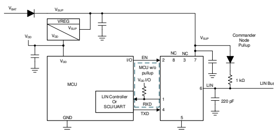
简化版原理图，指挥官模式
