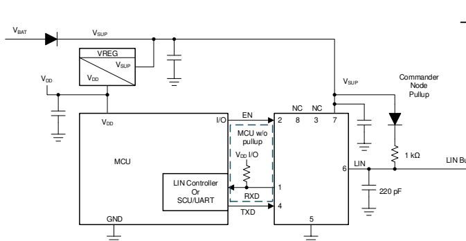
简化版原理图，指挥官模式
