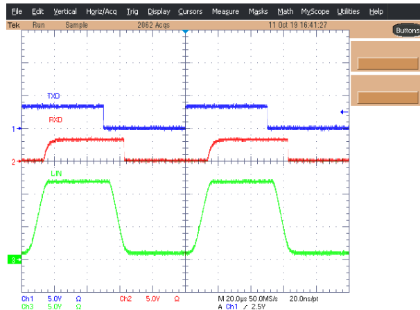
图 10-6. LIN Bus Performance
