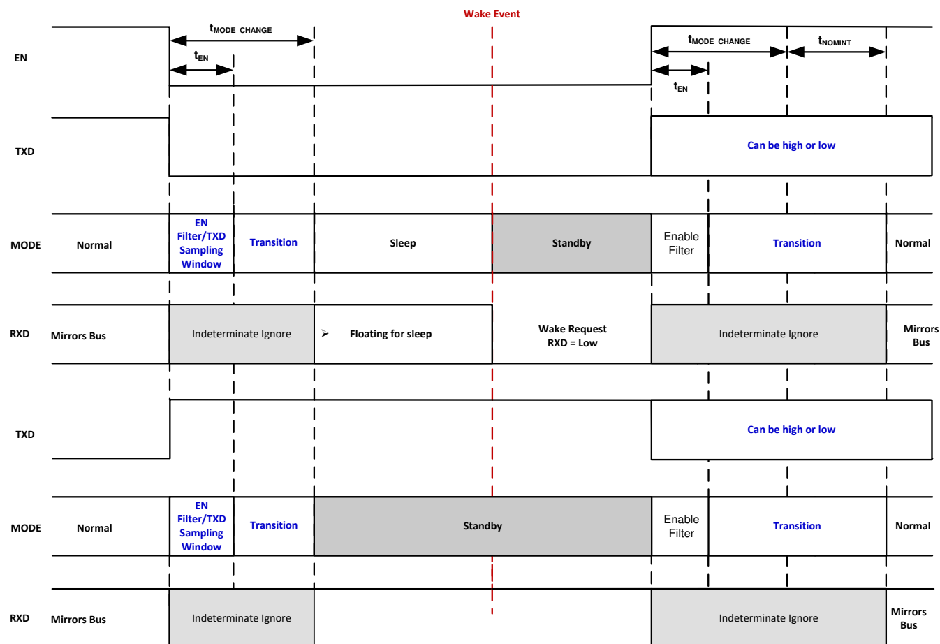
图 8-14. Mode Transitions
