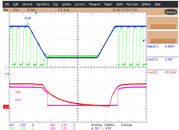
图 10-9. TLIN1028S-Q1 Brownout
