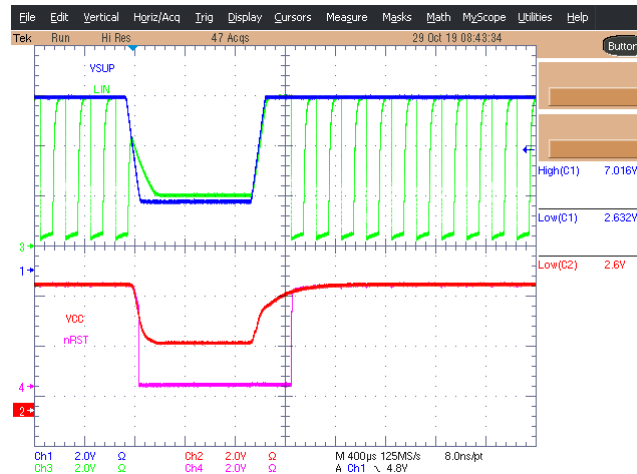
图 10-10. TLIN1028S-Q1 Brownout
