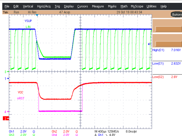
图 10-18. TLIN10285-Q1 Brownout
