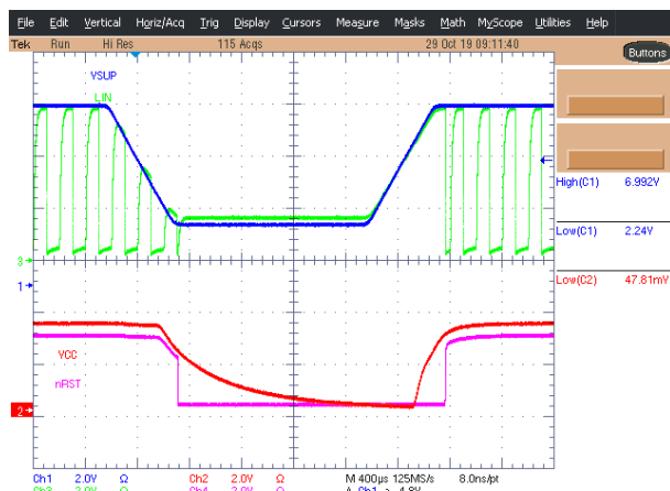
图 10-17. TLIN10283-Q1 Brownout
