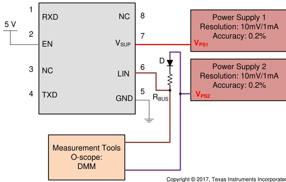
图 7-5. V_{SUP\_NON\_OP} Param 11
