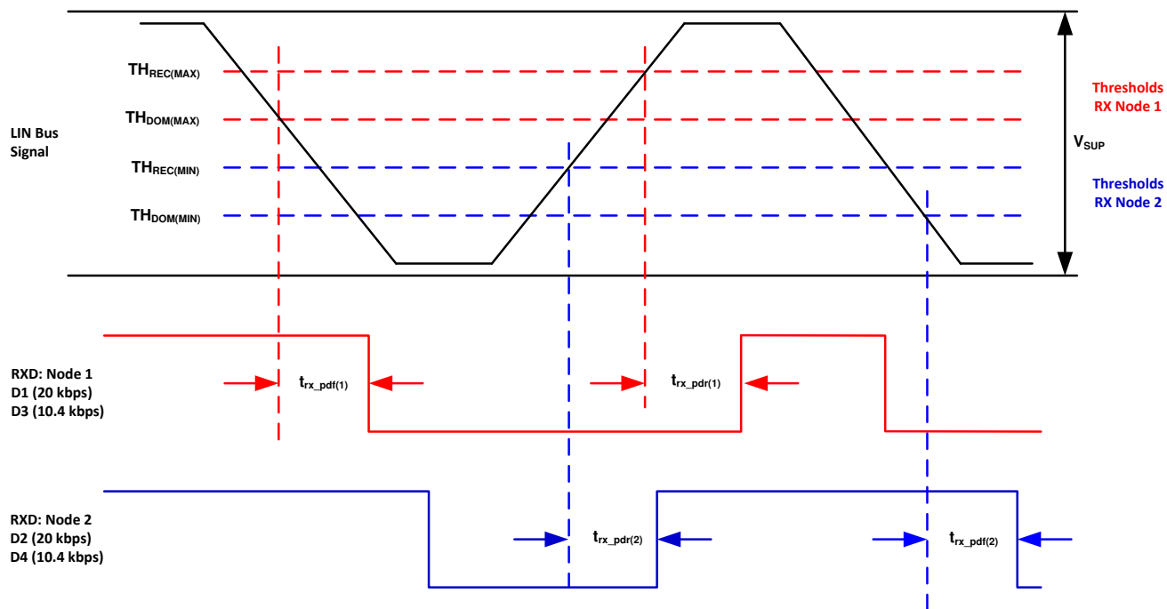
图 7-14. Propagation Delay
