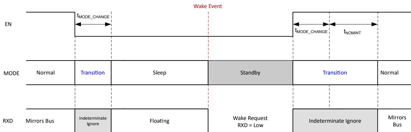
图 7-15. Mode Transitions
