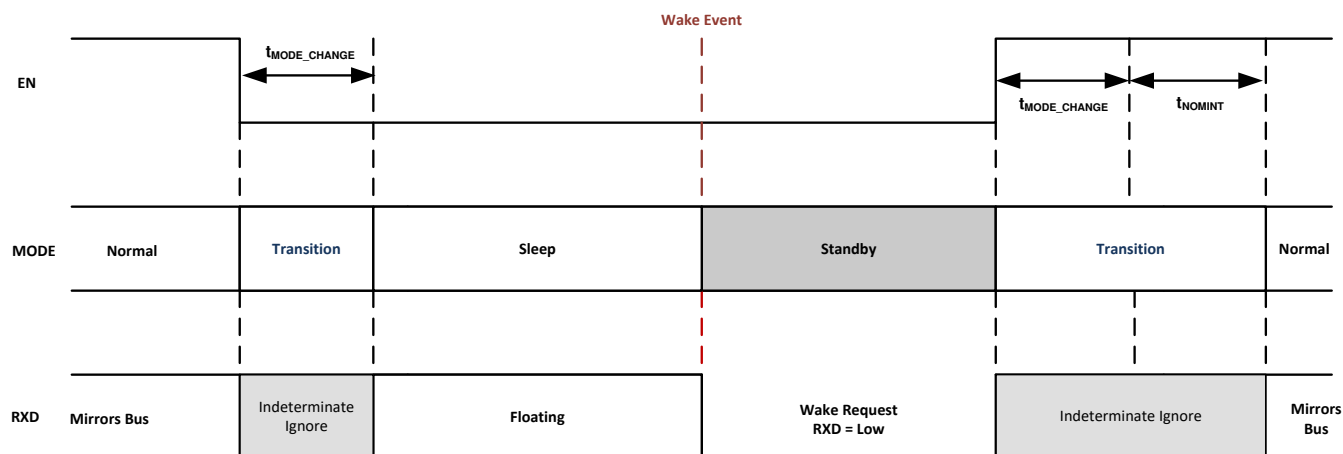
图 7-15. Mode Transitions
