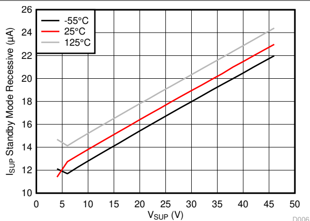
图 6-6. Standby Mode Recessive vs V_{SUP}
