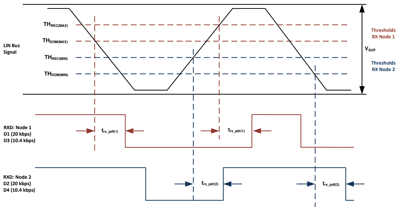
图 7-14. Propagation Delay
