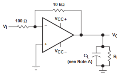
图 6-3. 单位增益带宽和相位裕度测试电路
