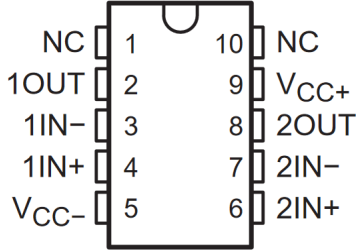
图 4-8. TLE2062 和 TLE2062A U 封装 ( 顶视图 )
