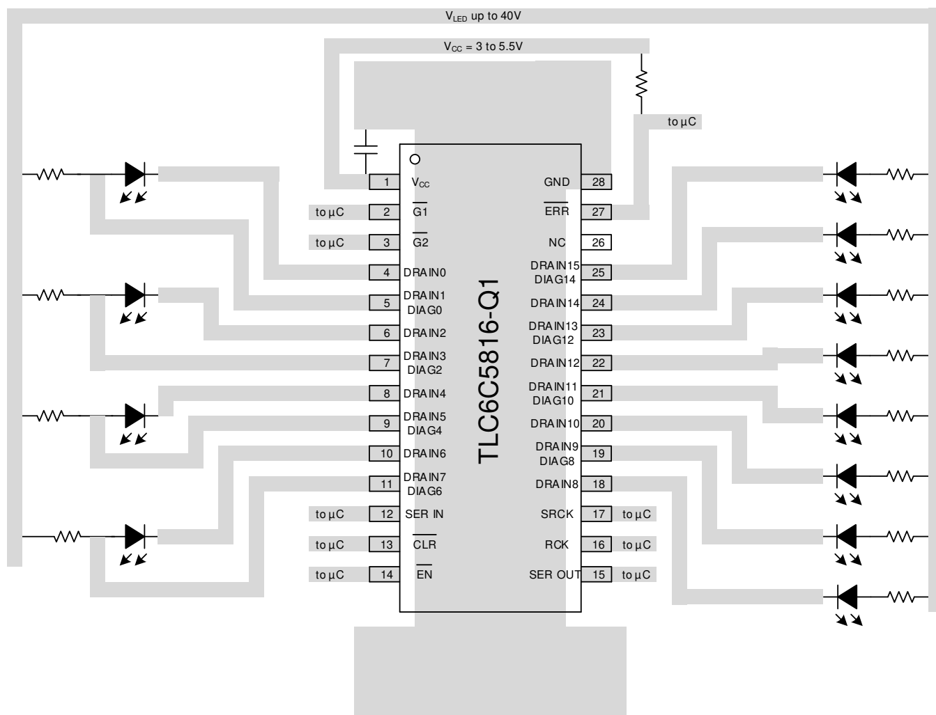
图 23. Layout Example
