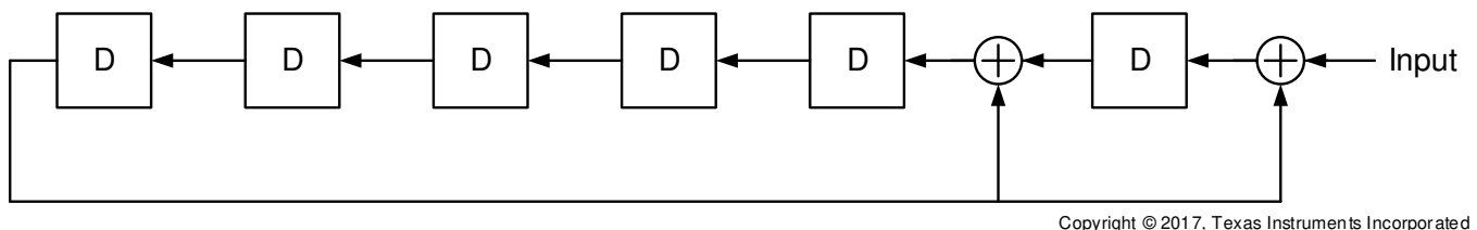
图 17. CRC Check Block Diagram
